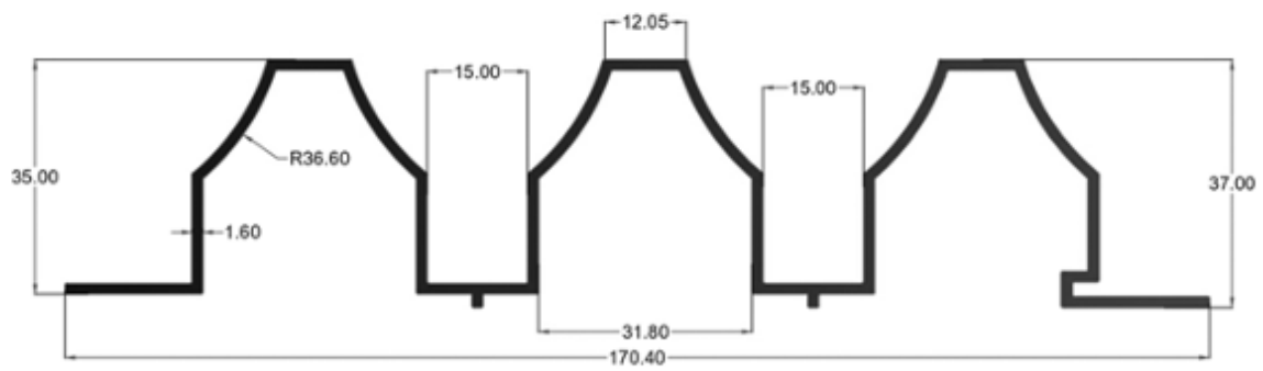
Section No : MCO 638( 3 BIG CONE) 5000GM / 12 FT
