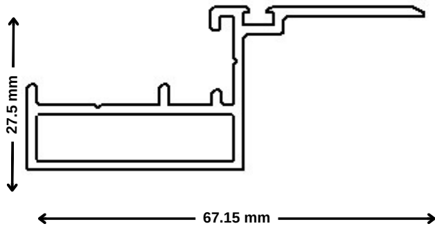
Interlock(101167)
