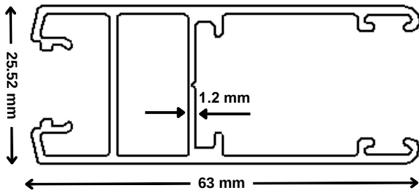
Shutter (101556)
