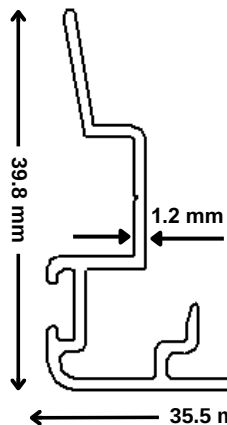
Interlock (101554)
