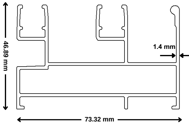
2 Track(101563)
